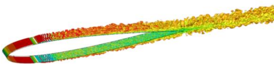
▲ Airfoil 전산유동해석 (현대중공업)
