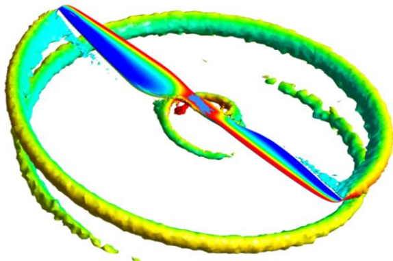
▲ 드론 프로펠러 공력해석 (항공우주연구원)
