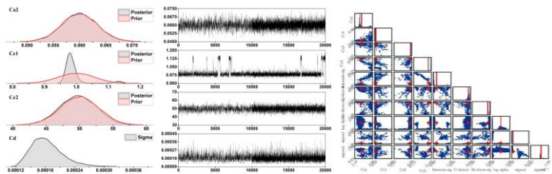
▲ CFD 해석 결과의 불확실성 정량화 (한국연구재단)
